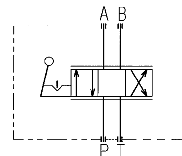
回 路 図
